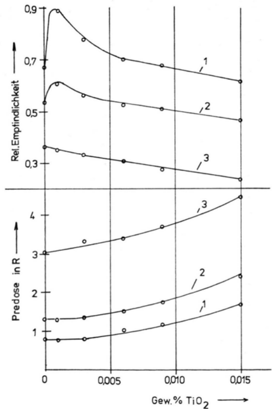
Abb. 1. Predose und Empfindlichkeit in Abhängigkeit der \text{TiO}_2 -Konzentration bei unterschiedlichen Ag-Konzentrationen (1): 3,6 Gew.-Proz.; (2): 6,9 Gew.-Proz.; (3): 10,3 Gew.-Proz. Ag.
